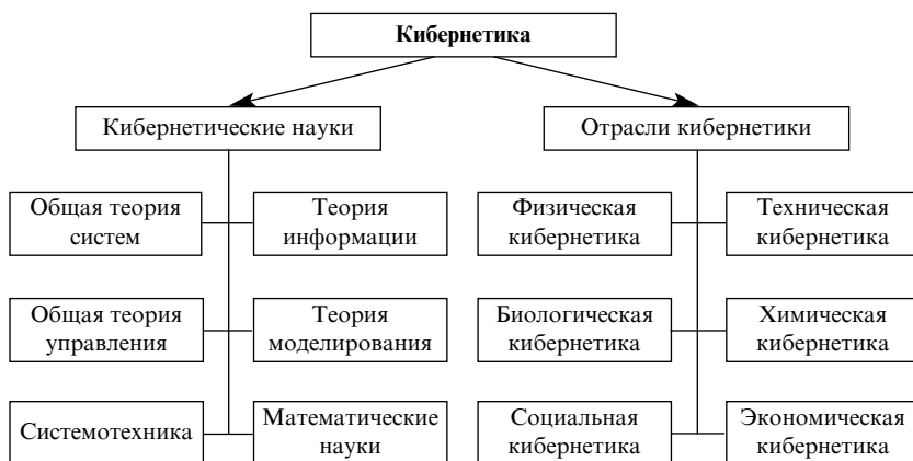
Рис. 21. Структура кибернетики
